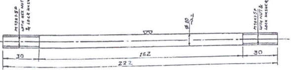
STUD. MAT:- EN-39 QTY:- 4 Nos.
