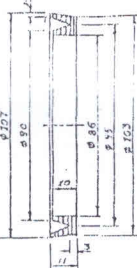
PISTON SLEEVE MAT:- NEOPRENE RUBBER. QTY:- 2 Nos. (SEPARATE DIAG NO:- M-2210-2)
