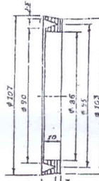
PISTON SLEEVE MAT: - NEOPRENE RUBBER. QTY: - 2 Nos. (SEPARATE DRG No: - M-2210-27)
