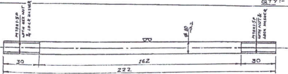
STUD. MAT: - EN-39 QTY: - 4 Nos.
